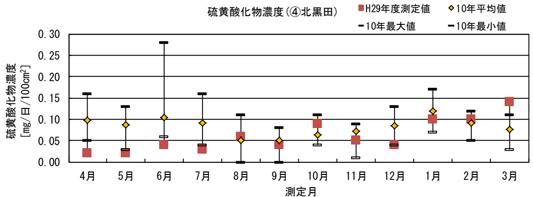
図 2-1 二酸化鉛法による硫酸化物濃度の比較結果
