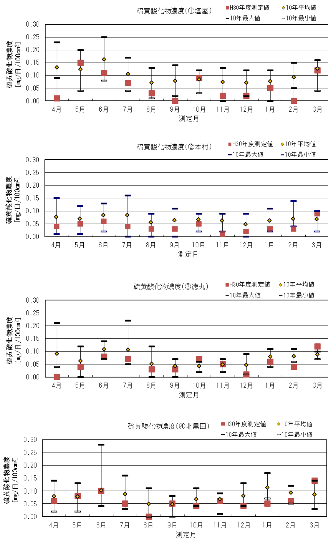
図 2-1 二酸化鉛法による硫黄酸化物濃度の比較結果
