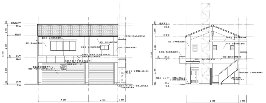
第9分団消防詰所設計図(立面図)より
