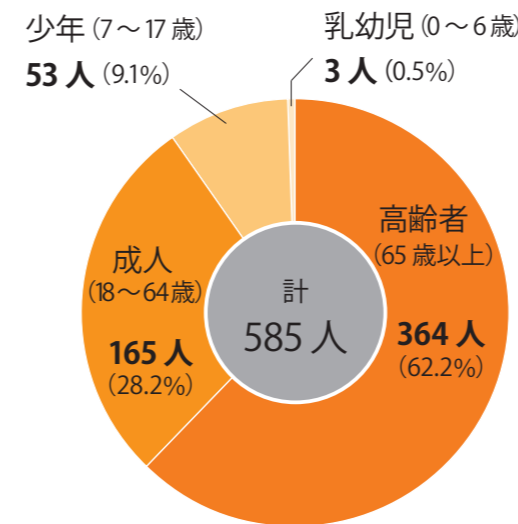
熱中症による救急搬送人員数の年齢別割合 (愛媛県R3)
