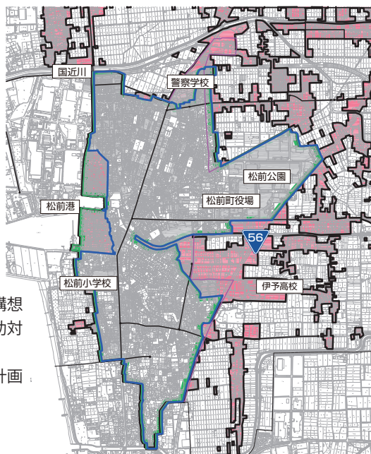
▼公共下水道整備構想図
