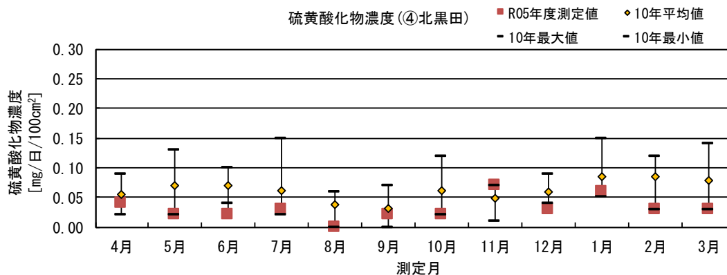
図 2-1 二酸化鉛法による硫黄酸化物濃度の比較結果
