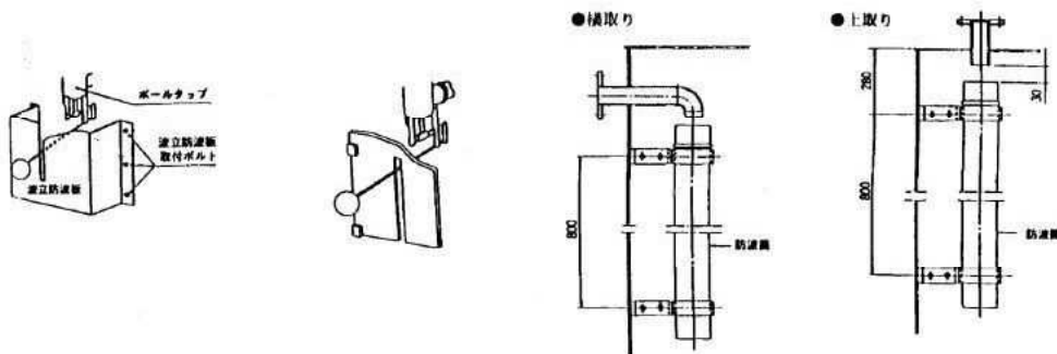
図 5-1 波立ち防止装置設置例
