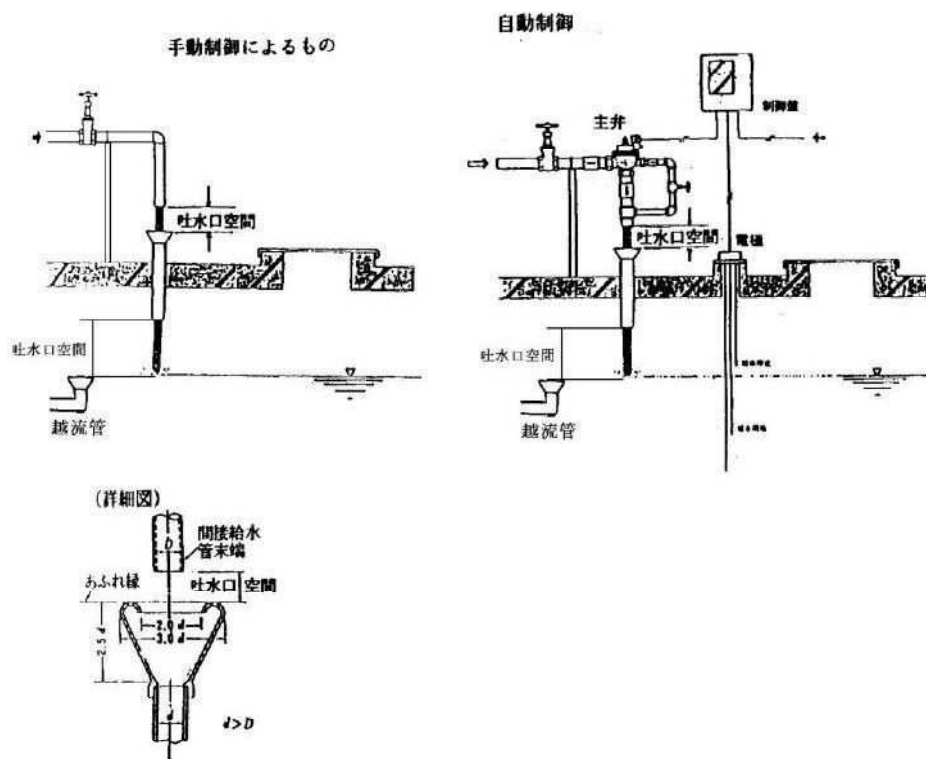
図4 二重の吐水口空間の確保
