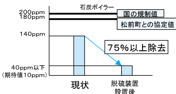
図2 脱硫装置の設置前後の排出状況(煤じん)
